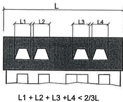
Bild 1: Schema Dachaufbauten
